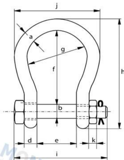
Třmen omega s maticí široký G-4263 Green Pin
